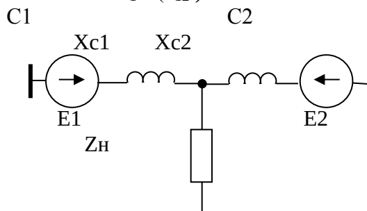
Рис. 3 Схема замещения электропередачи для расчета действительного предела мощности при нагрузке Z_H , заданной постоянным сопротивлением
